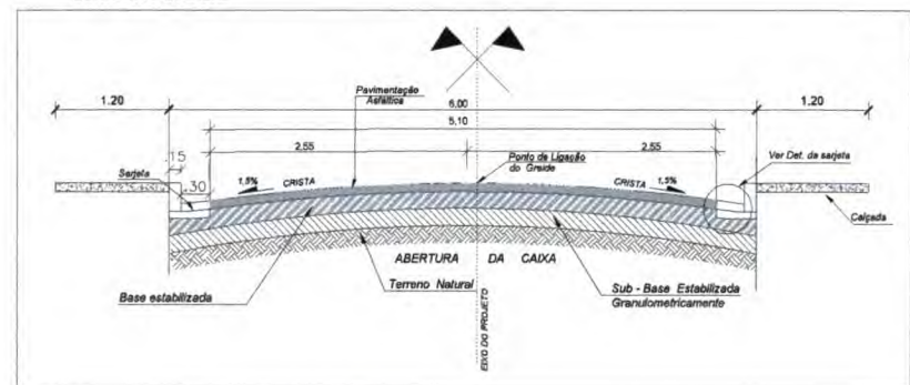
CORTE TRANSVERSAL
