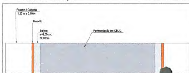
DETALHE DA PAVIMENTAÇÃO
