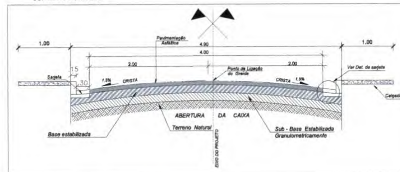
CORTE TRANSVERSAL
