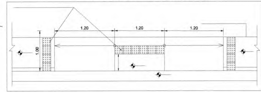
DETALHE DA ACESSIBILIDADE - CALÇADA COM LARGURA DE 1,00 M (CADA LADO)
