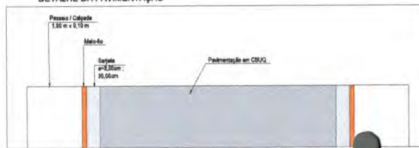
DETALHE DA PAVIMENTAÇÃO
