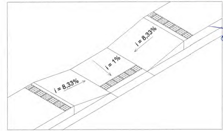
PESPECTIVA DA RAMPA
