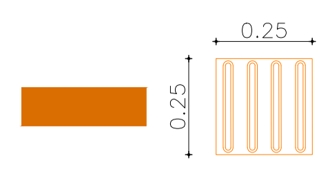
Sinalização tátil de direção - Modulação do piso
