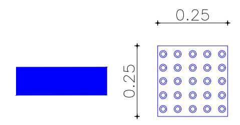
Sinalização tátil de alerta - Modulação do piso
