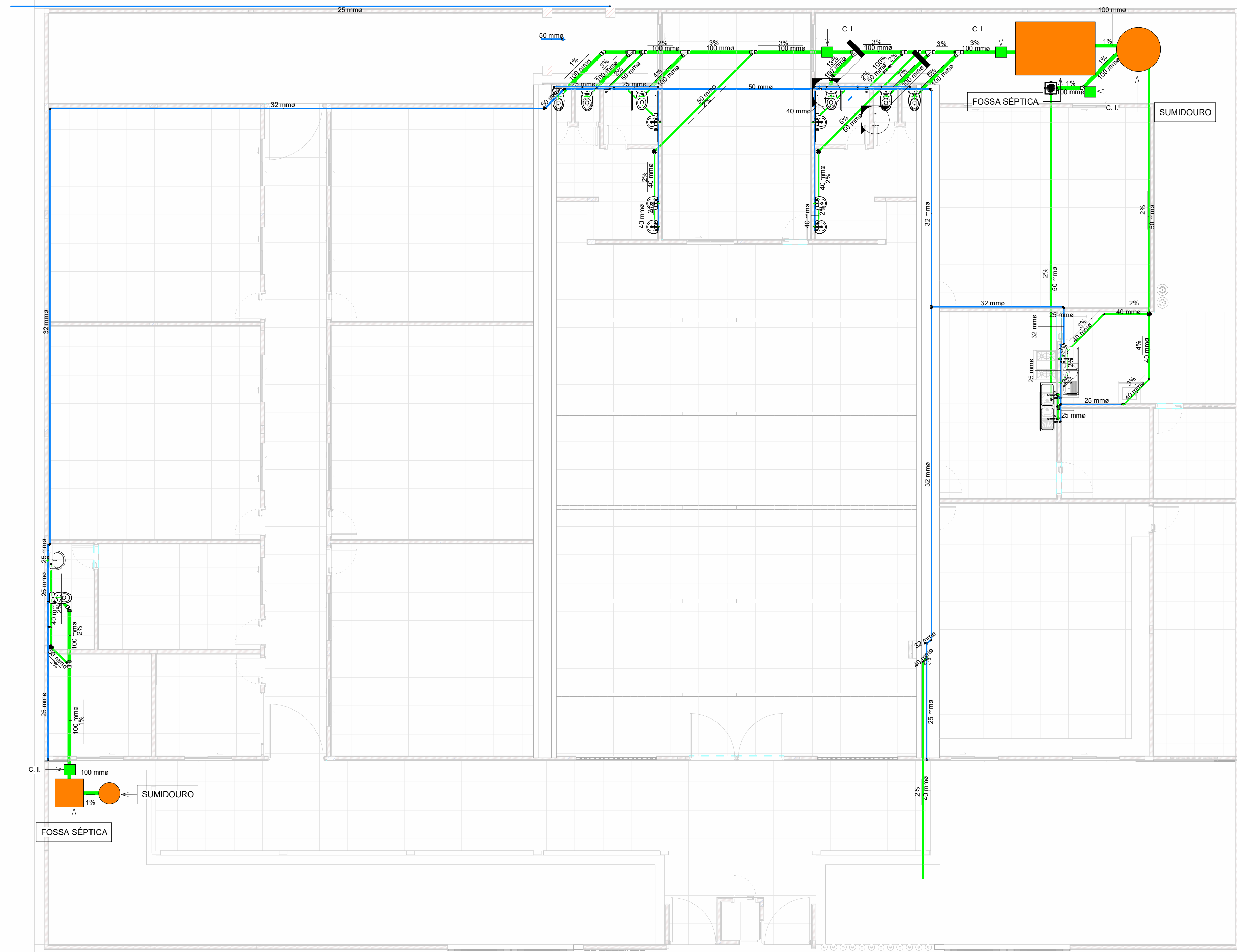
PLANTA BAIXA GERAL ESCALA 1/75
