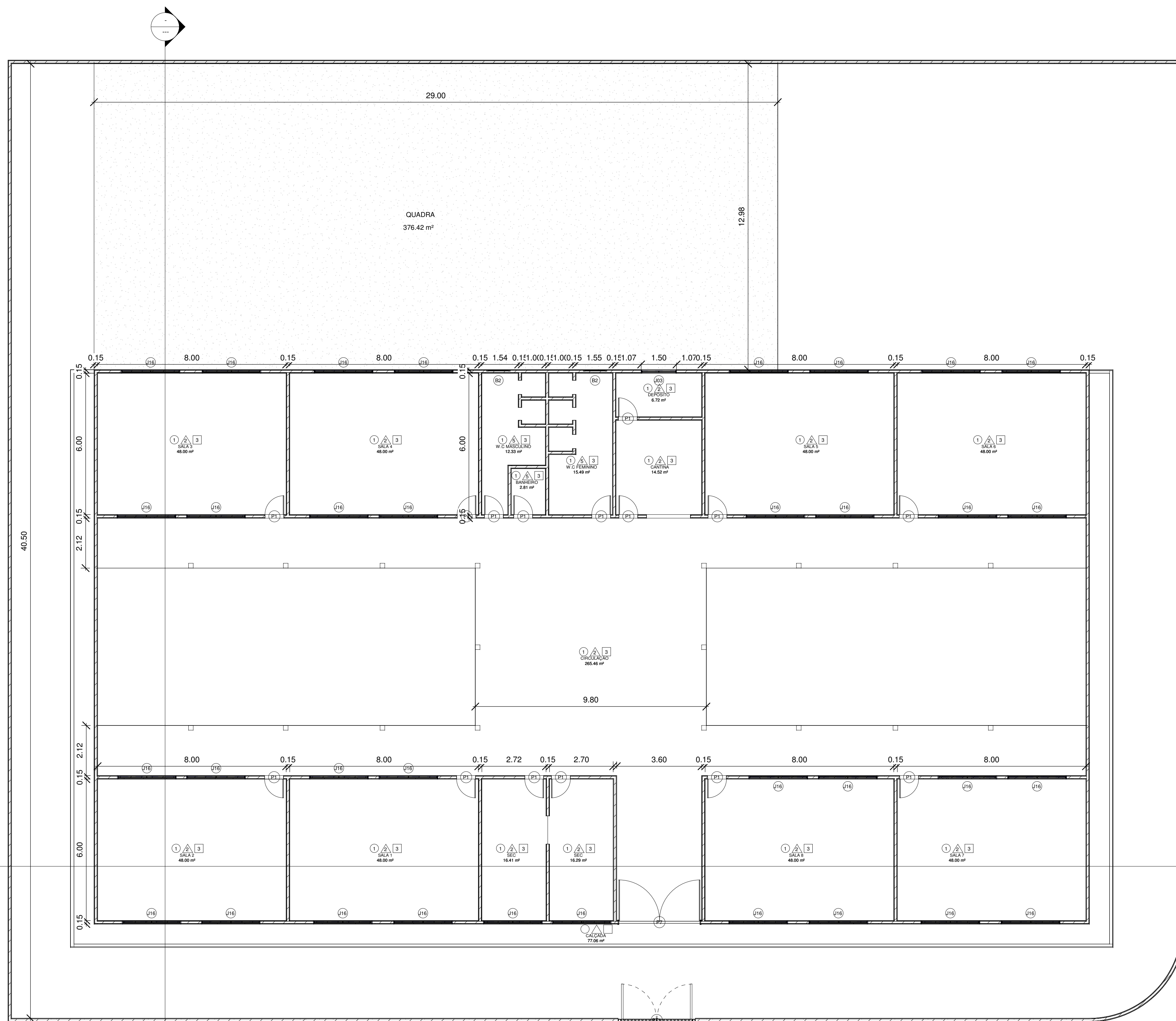
1 PLANTA BAIXA 1 : 100
